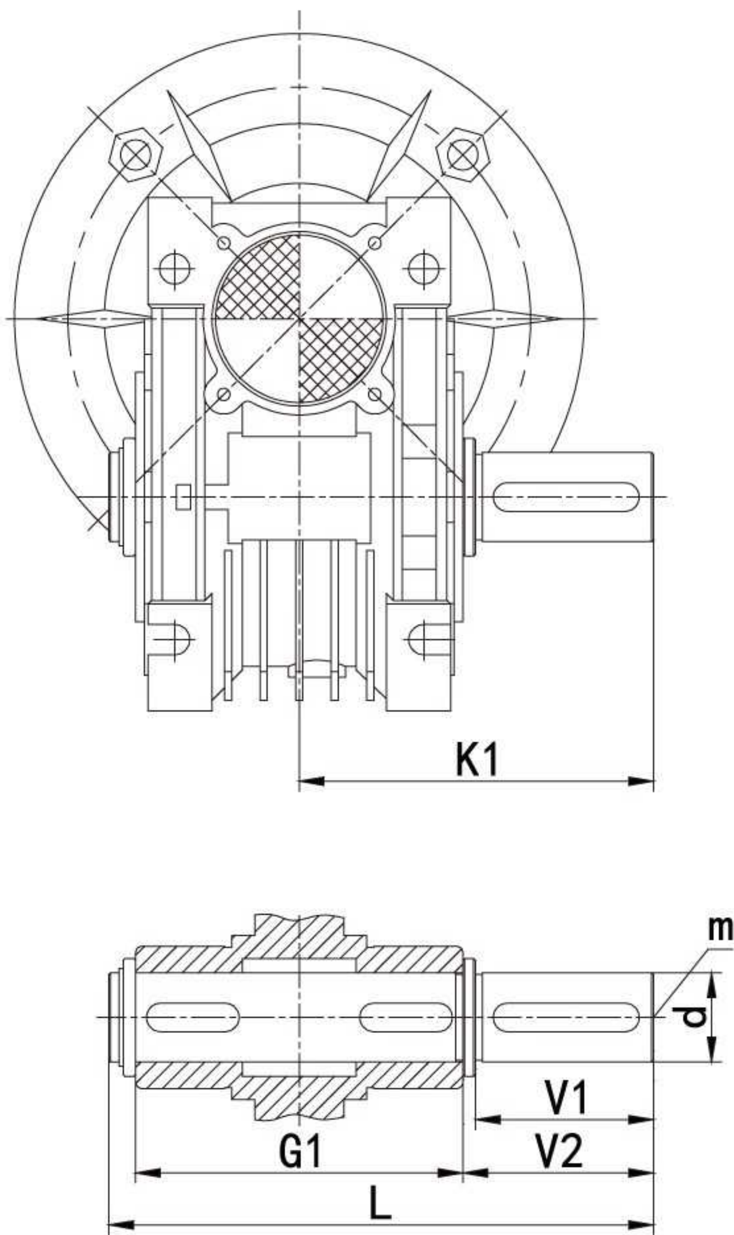
单向输出轴 (DZ)
