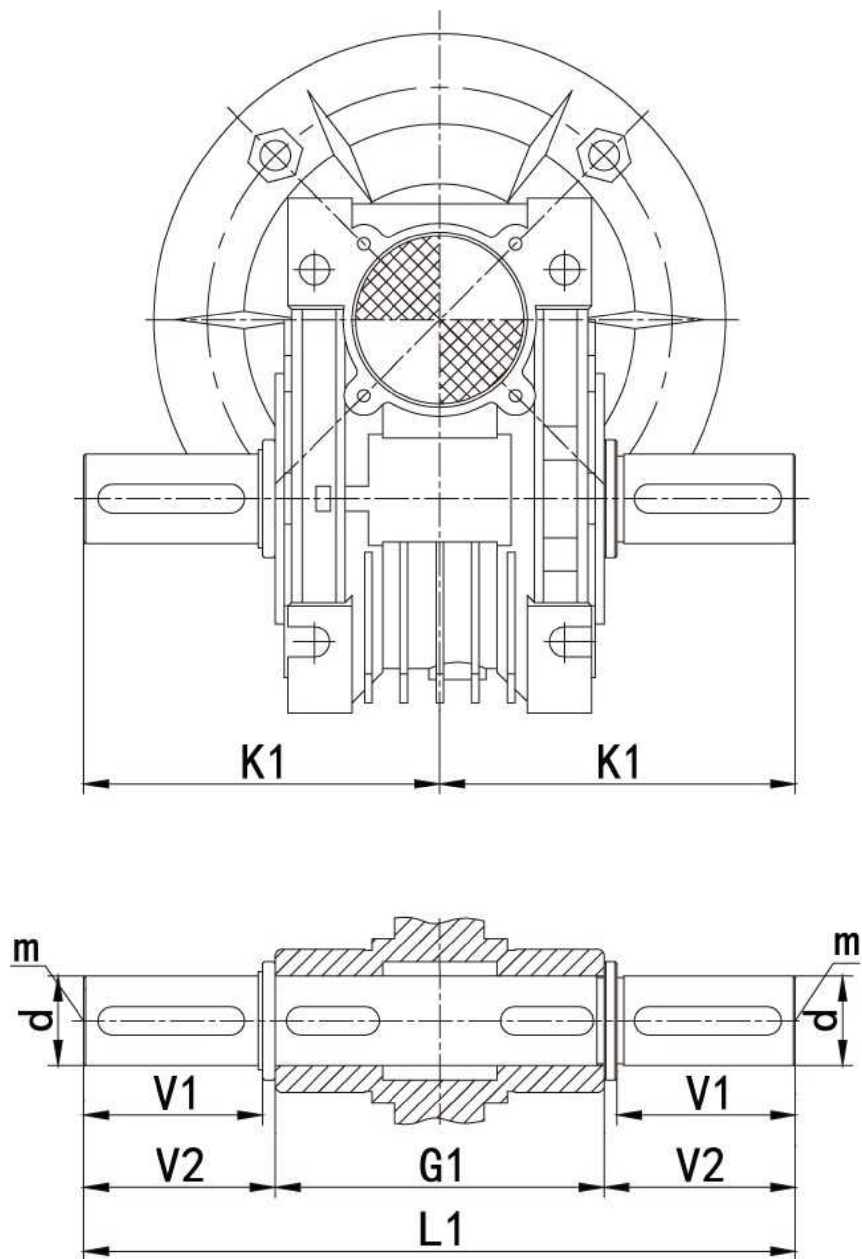
双向输出轴 (SZ)
